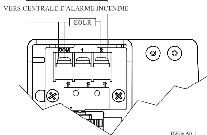
Raccordement du signal basse pression Fig. 4
